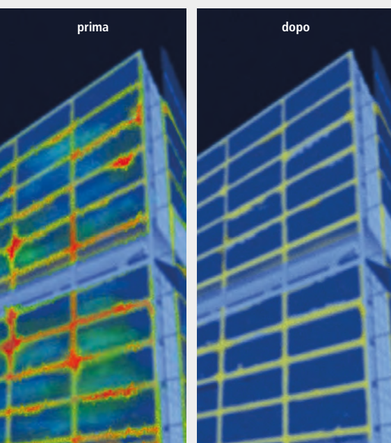
Immagine della dissipazione di calore di un edificio prima e dopo.
